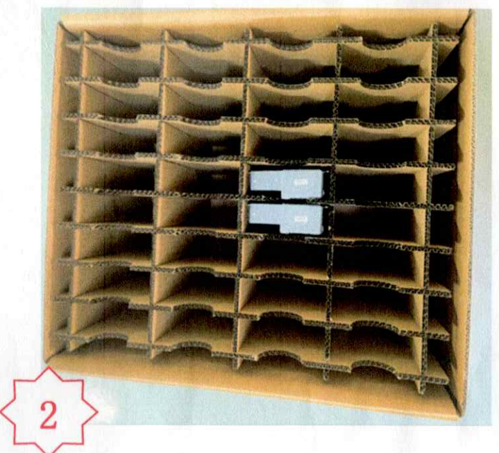
图二，将 9 个长刀卡和 5 个短刀卡如图所示进行组装，一箱一层，一层 32PCS。
